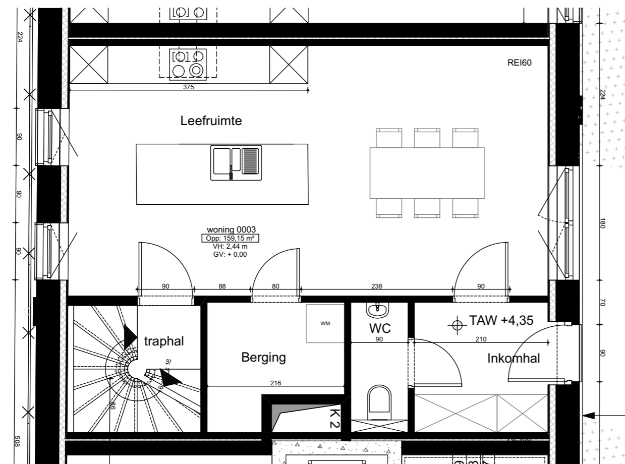
GELIJKVLOERS
