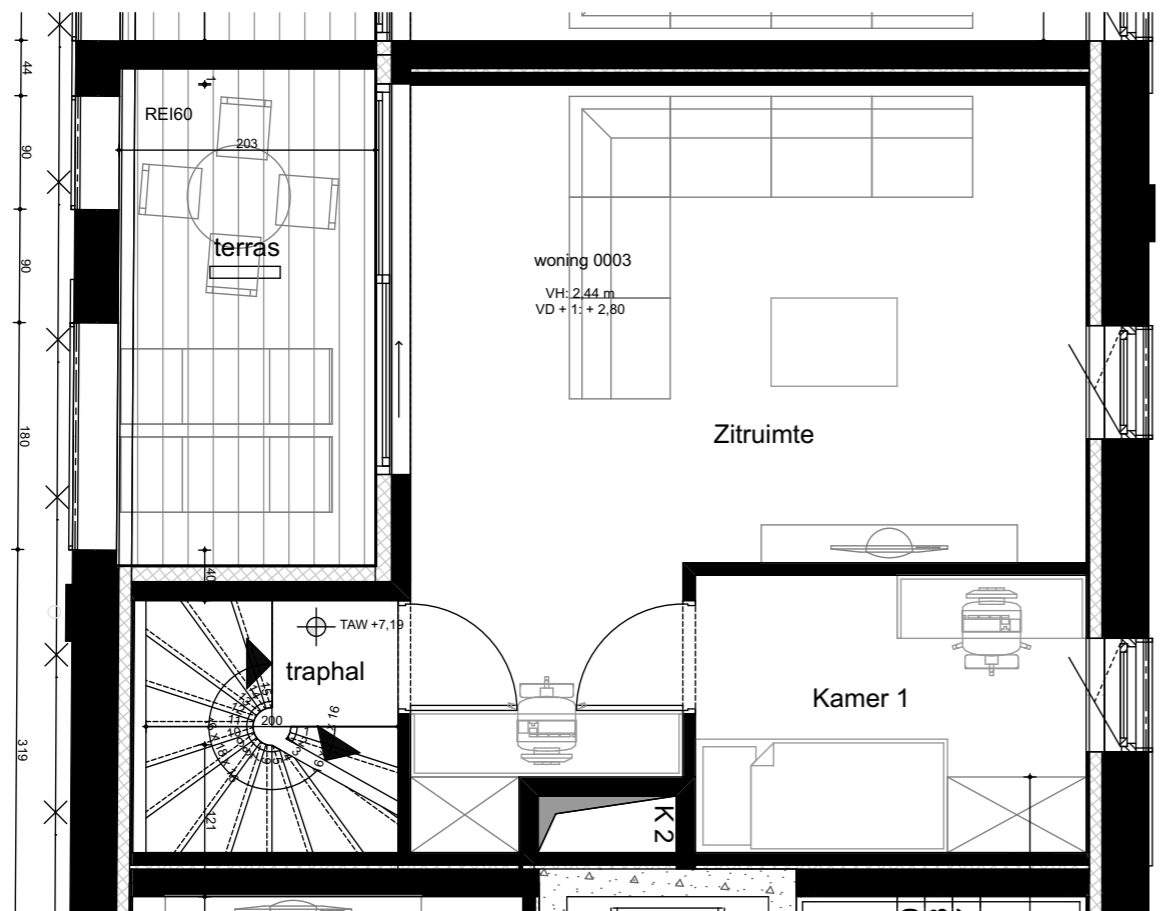
1ste VERDIEPING
