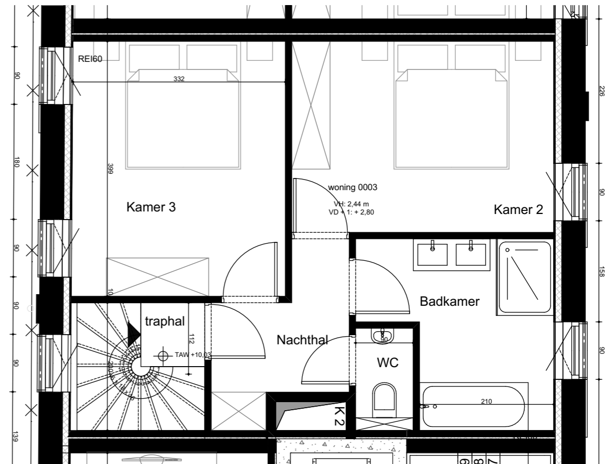
2de VERDIEPING
