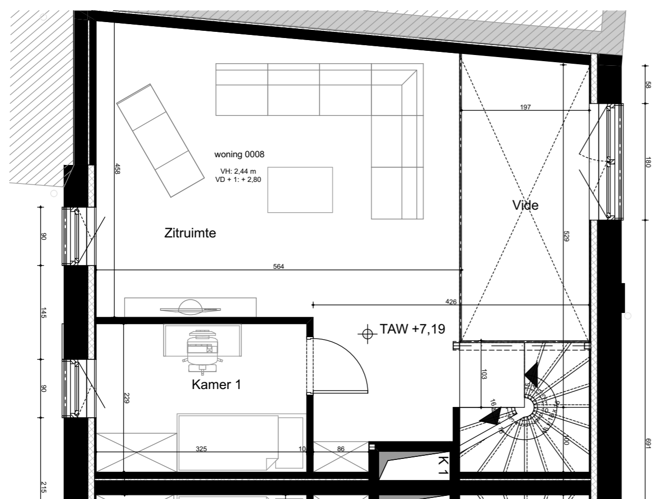
1ste VERDIEPING
