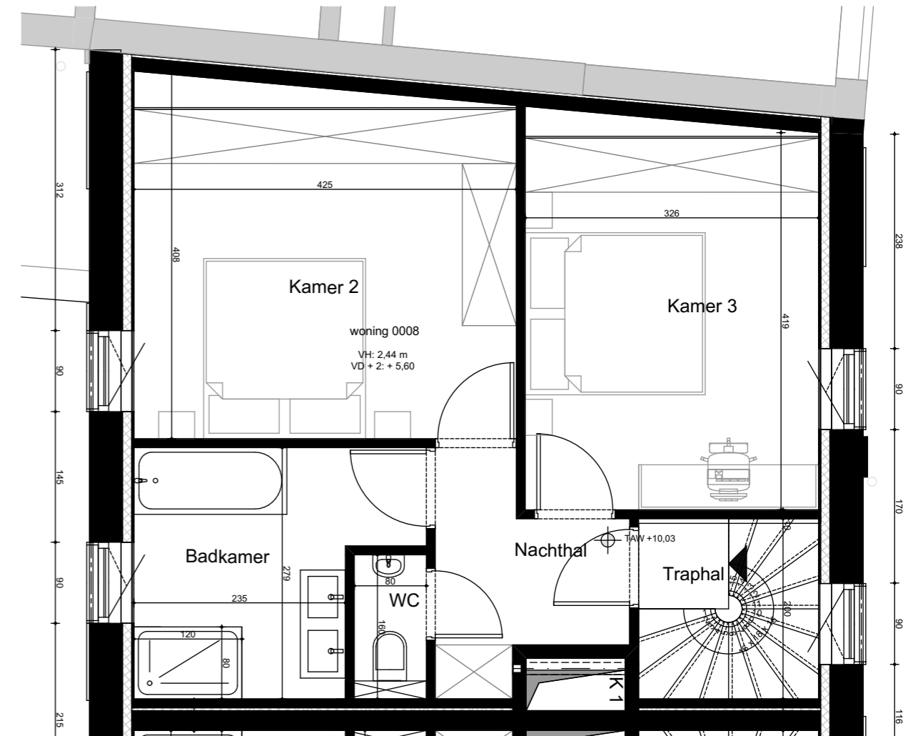
2de VERDIEPING
